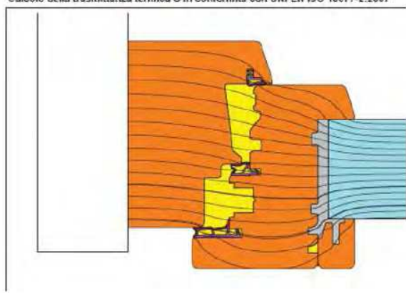
Calcolo della trasmittanza termica U in conformità con UNI EN ISO 10077-2:2007
